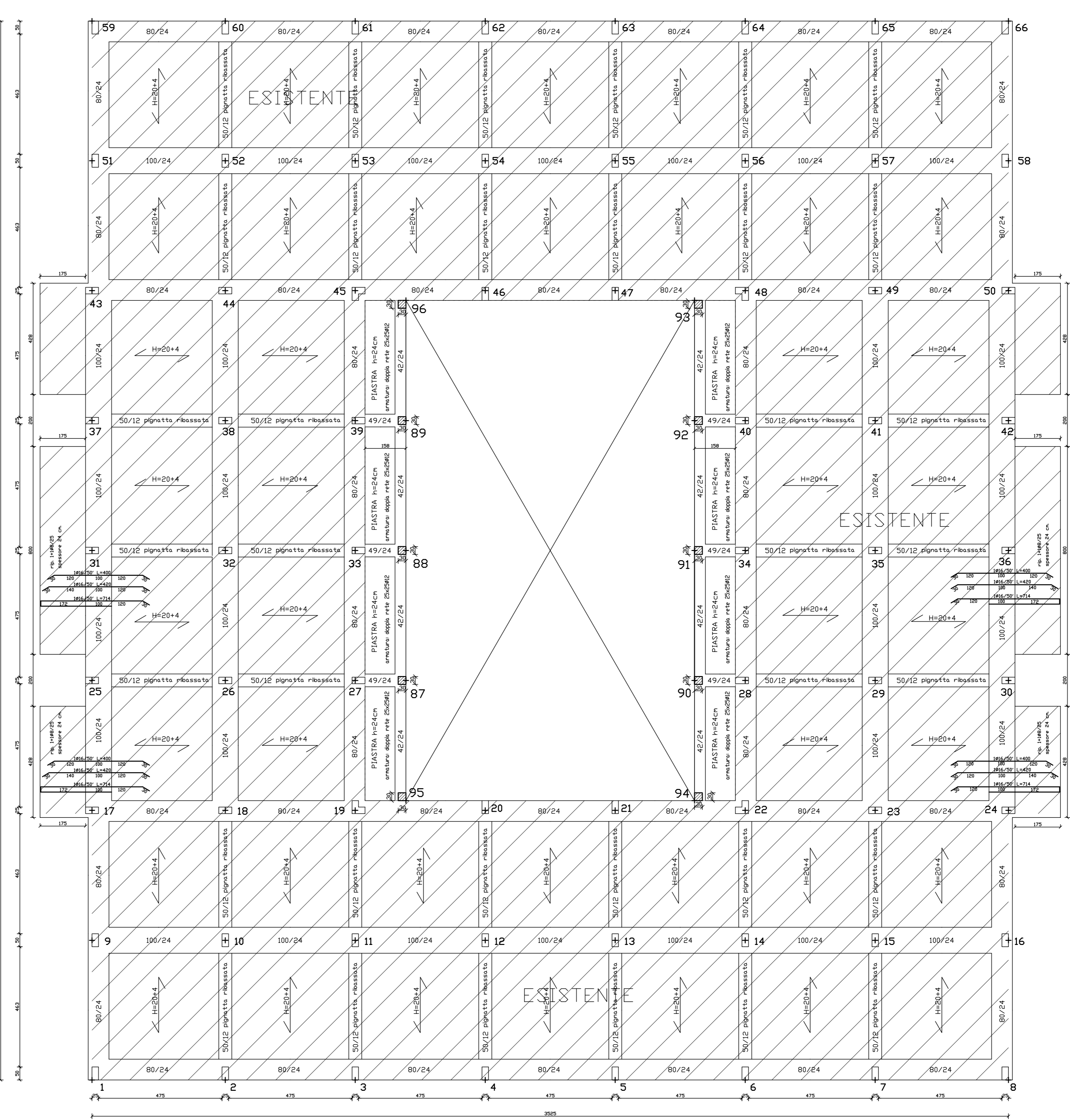
CARPENTERIA SOLAIO QUOTA m: 3.25
