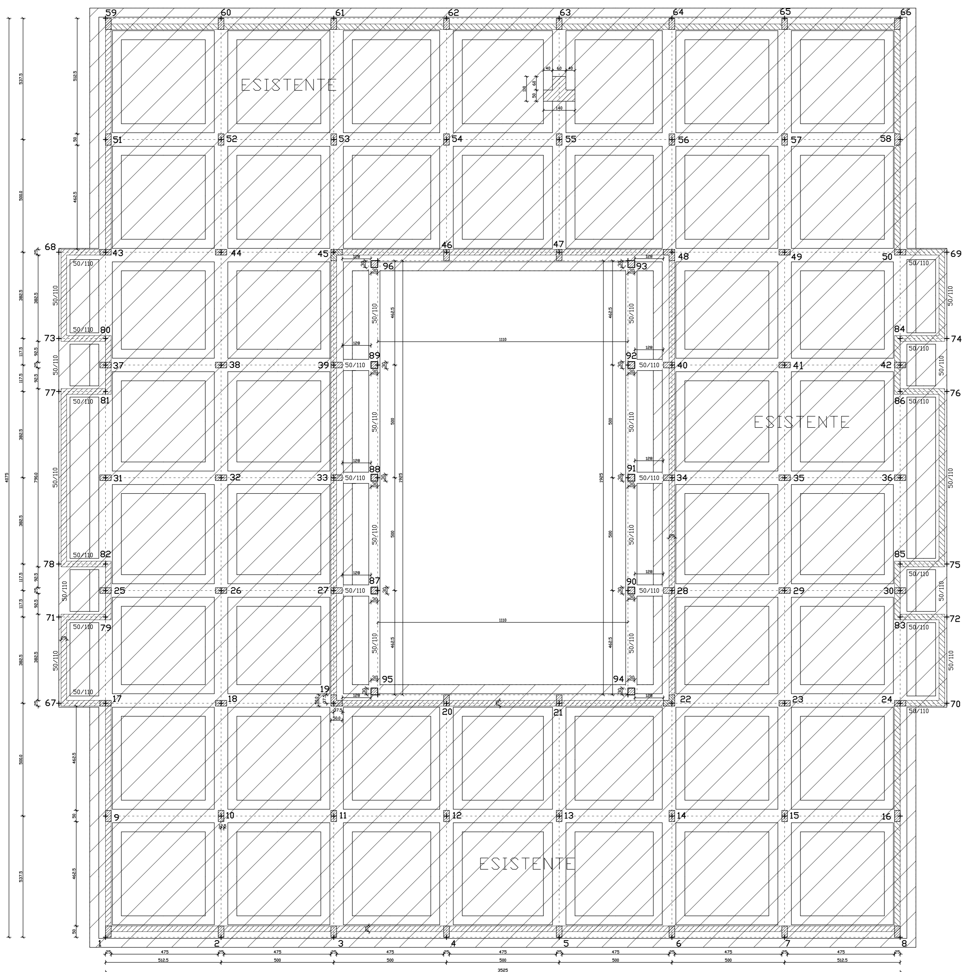
CARPENTERIA FONDAZIONI QUOTA m 0.00
