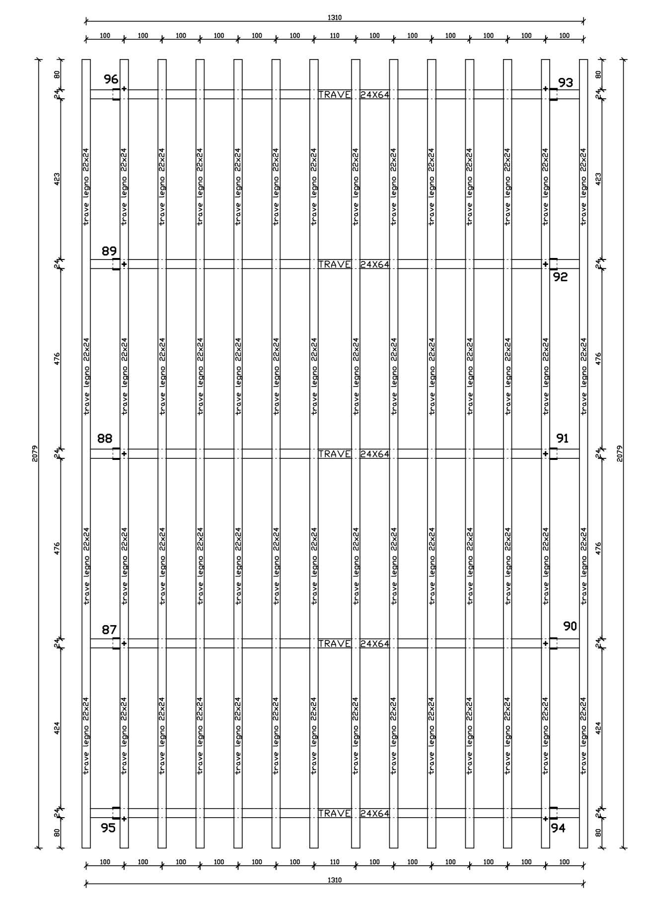
CARPENTERIA COPERTURA QUOTA m: 5.20
